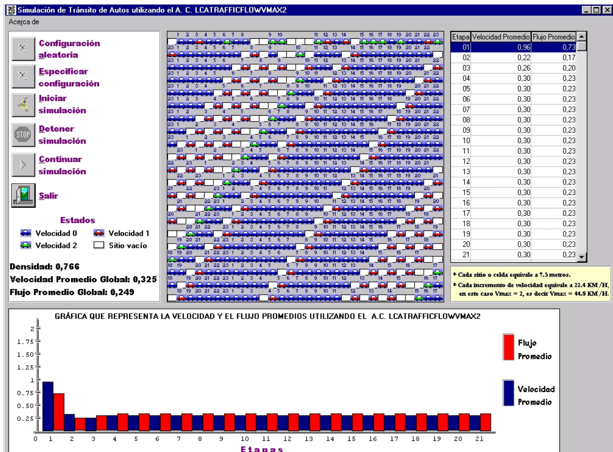
Figura 6.4: Pantalla donde se muestra la evolución del autómata con un arreglo pequeño.
