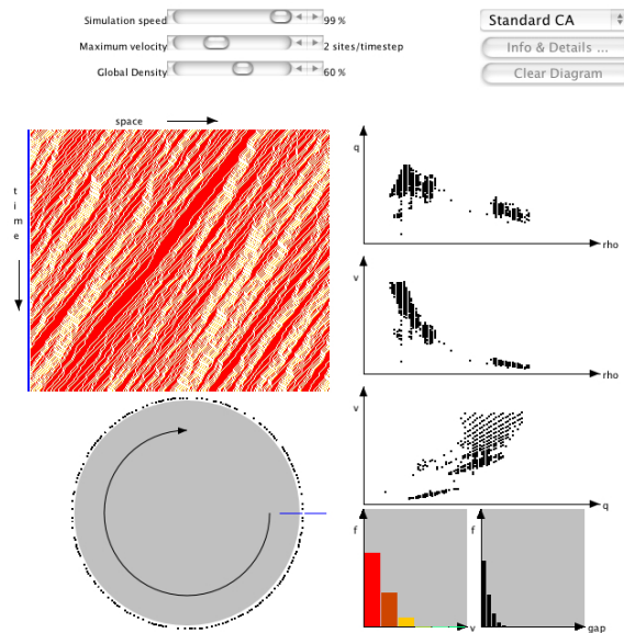
Figura 2.2: Simulación disponible en [76]
