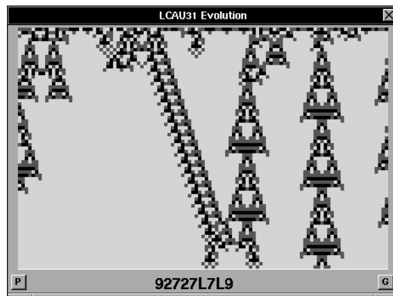
Figura 3.17: Diagrama de evoluciones de un autómata celular lineal (3,1) aplicando la regla 92727L7L9.
