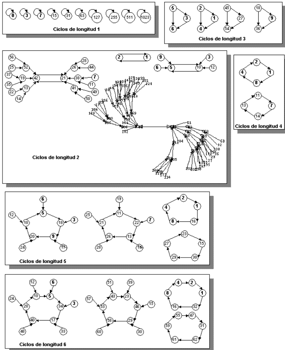
Figura 4.14: Ciclos de periodo 1 a periodo 6 de la regla 184.
