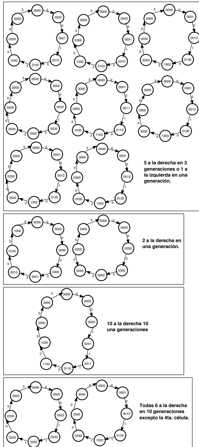
Figura 5.13: Anillos que generan secuencias en las cuales las células tienen desplazamientos uniformes hacia la derecha.
