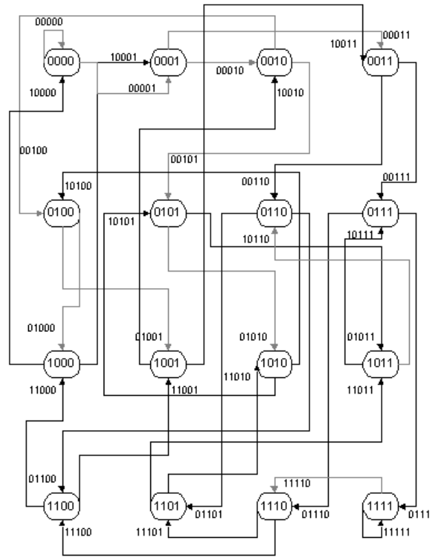
Figura 4.11: Diagrama de Bruijn extendido a vecindades parciales de 4 células.
