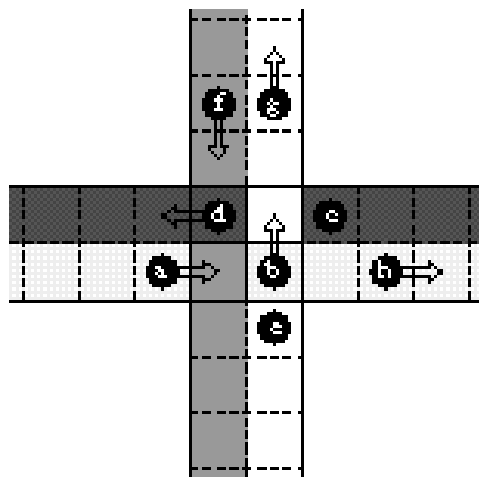
Figura 2.4: Ejemplo de una configuración cerca de un cruce. Las cuatro celdas centrales representan una rotación la cual está desplazándose en sentido opuesto a las manecillas del reloj. Los diferentes tonos de color gris junto con el color blanco indican las diferentes direcciones que siguen los carriles de tránsito indicadas por las flechas. Los puntos etiquetados con letras son los autos, que pueden moverse hacia la dirección indicada por la flecha. Los autos sin una flecha no tienen permitido moverse.
