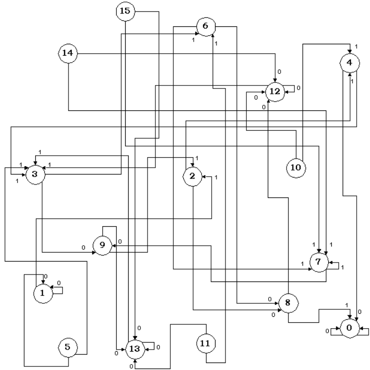
Figura 3.25: Diagrama de subconjuntos de la regla 54.
