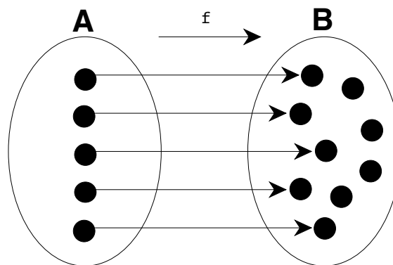
Figura 3.20: Función inyectiva.
