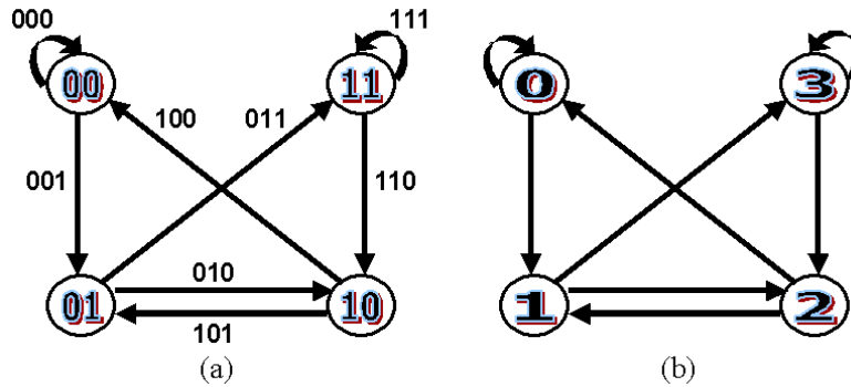
Figura 3.23: Diagramas de Bruijn genéricos para un autómata celular lineal (2,1). En el diagrama del lado izquierdo (a) las vecindades parciales están expresadas en notación binaria, mientras que en el diagrama del lado derecho (b) están en notación decimal.
