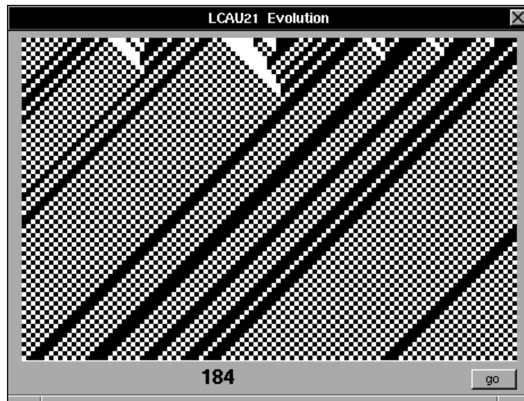
Figura 4.17: Simulación del flujo de tránsito representada mediante el diagrama de evoluciones.
