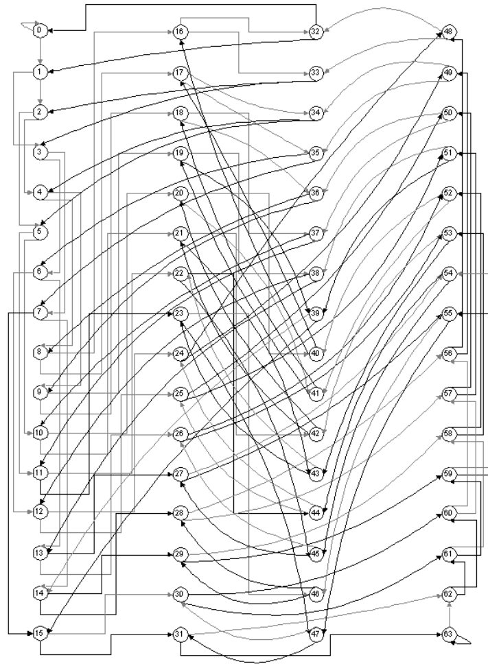
Figura 4.12: Diagrama de Bruijn extendido a vecindades parciales de 6 células.
