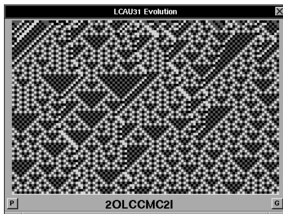
Figura 3.16: Diagrama de evoluciones de un autómata celular lineal (3,1) aplicando la regla 2OLCCMC2I.
