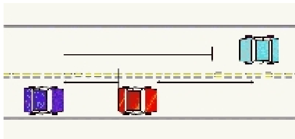
Figura 2.3: Modelo bi-direccional para flujo de tránsito.
