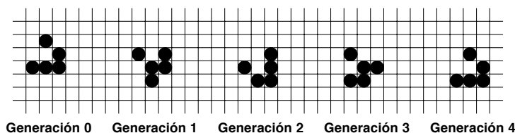
Figura 3.5: Uno de los descubrimientos de Conway más remarcable es la figura formada por cinco células vivas llamada glider . Después de transcurridas dos generaciones, el glider tiene un ligero acarreo hacia la derecha, el cual se ve reflejado en una línea diagonal. A este fenómeno se le conoce como “ glide reflection ” debido al nombre de la figura. Una vez que transcurren dos generaciones más, el glider se endereza a sí mismo y entonces se ha movido en la cuadrícula un lugar diagonalmente hacia abajo y a la derecha desde su posición inicial.
