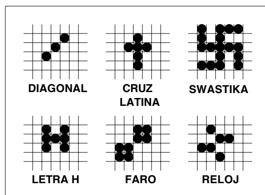
Figura 3.4: Configuraciones en las que todas la células vivas mueren.
