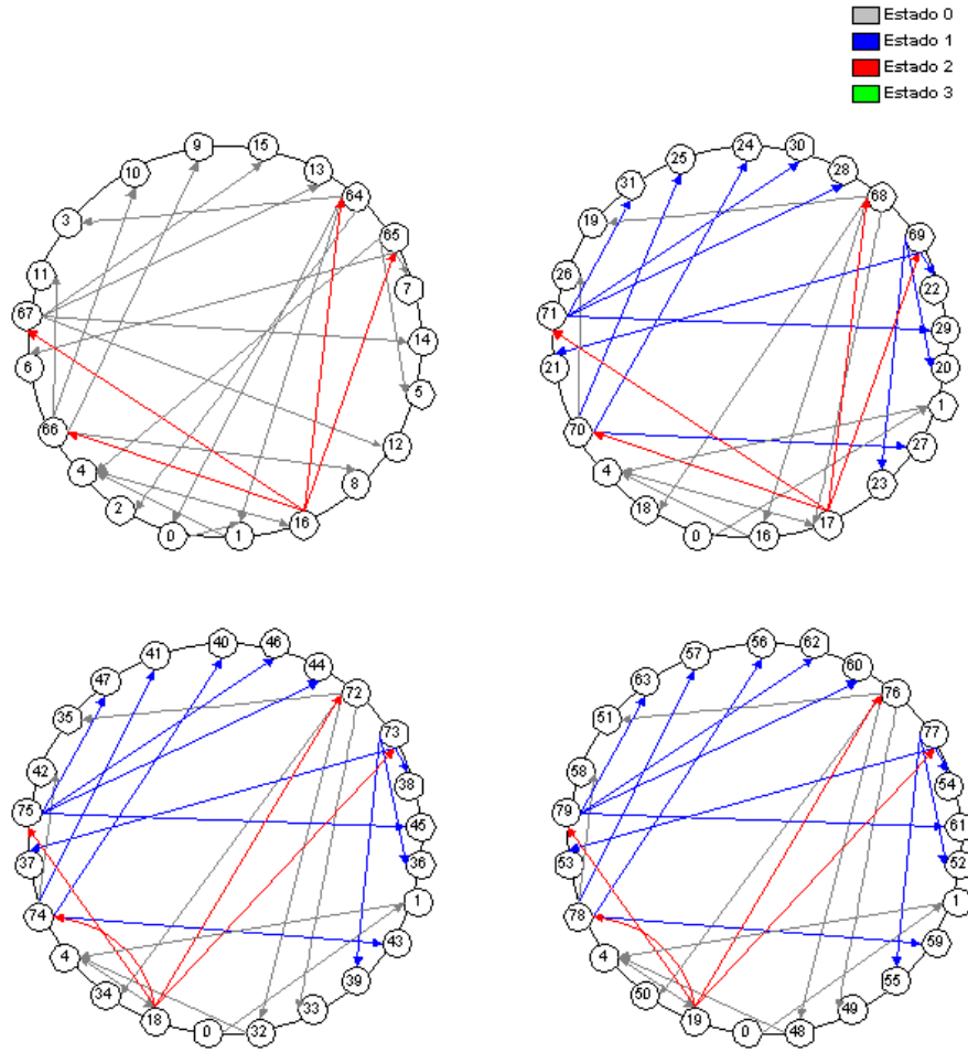
Figura 5.10: Fragmento del diagrama de Bruijn de LCATRAFFICFLOWVMAX2 el cual tiene un comportamiento equivalente al del modelo de Nagel con V_{max} = 2 .
