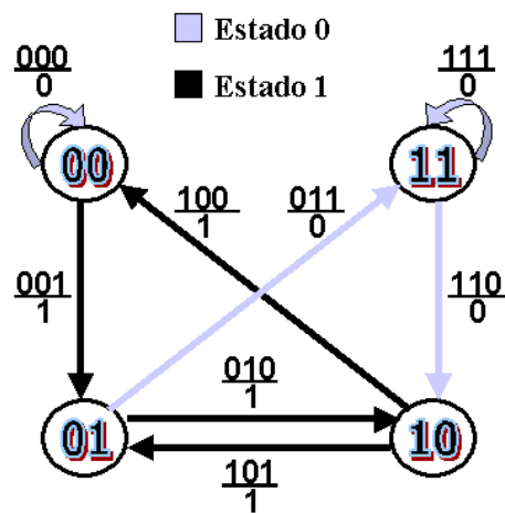
Figura 3.24: Diagrama de Bruijn de la regla 54.
