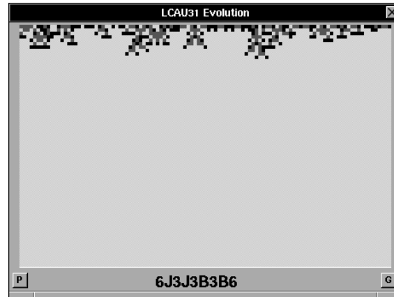
Figura 3.14: Diagrama de evoluciones de un autómata celular lineal (3,1) aplicando la regla 6J3J3B3B6.
