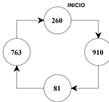
Figura 3.19: Ciclo de periodo 4.
