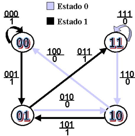
Figura 5.4: Diagrama de Bruijn de la regla 43.
