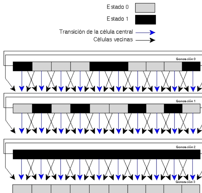
Figura 3.12: Transiciones globales de un autómata celular lineal (2,1) aplicando la regla 54.
