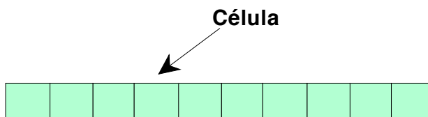
Figura 3.6: Arreglo de 10 células.
