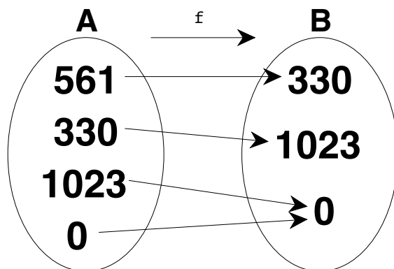
Figura 3.13: Función de transiciones globales aplicando la regla 54.
