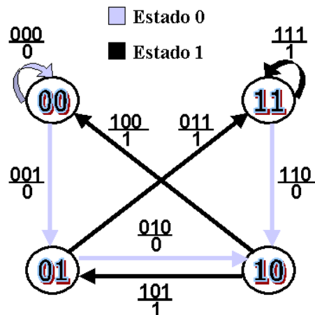
Figura 4.8: Diagrama de Bruijn de la regla 184.
