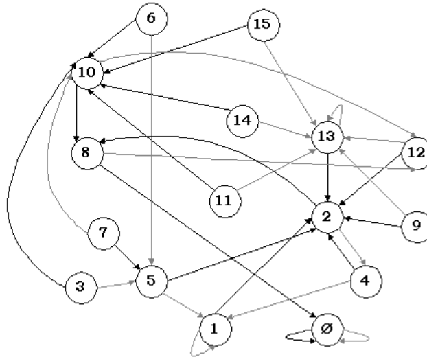
Figura 5.5: Diagrama de subconjuntos de la regla 43.
