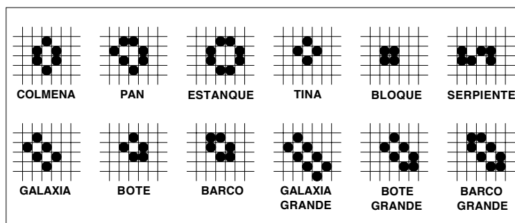
Figura 3.3: A las configuraciones que permanecen estables durante toda la evolución del autómata celular se les conoce como still life .
