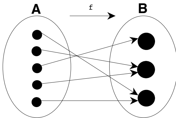
Figura 3.21: Función sobreyectiva.
