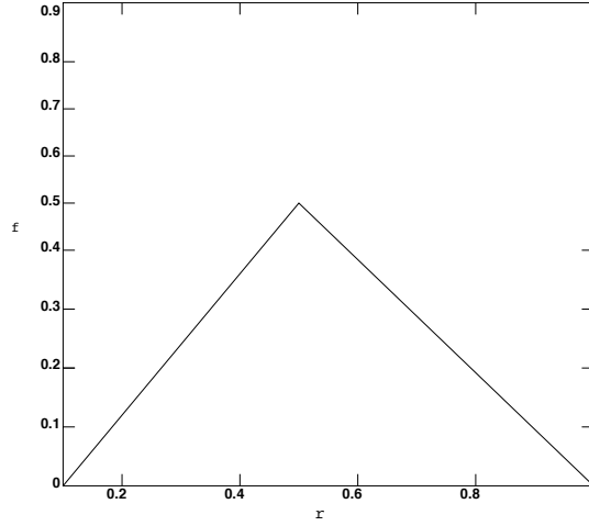
Figura 4.6: Diagrama fundamental de la regla 184.
