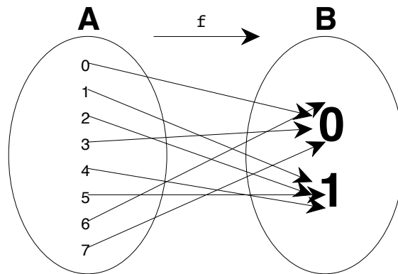
Figura 3.9: Función de transiciones locales de la regla 54.
