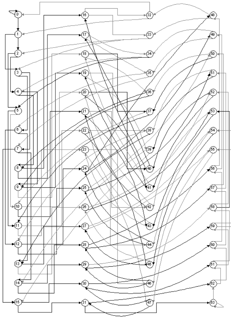
Figura 5.7: Diagrama de Bruijn de la regla 43 extendido a vecindades parciales de 6 células.
