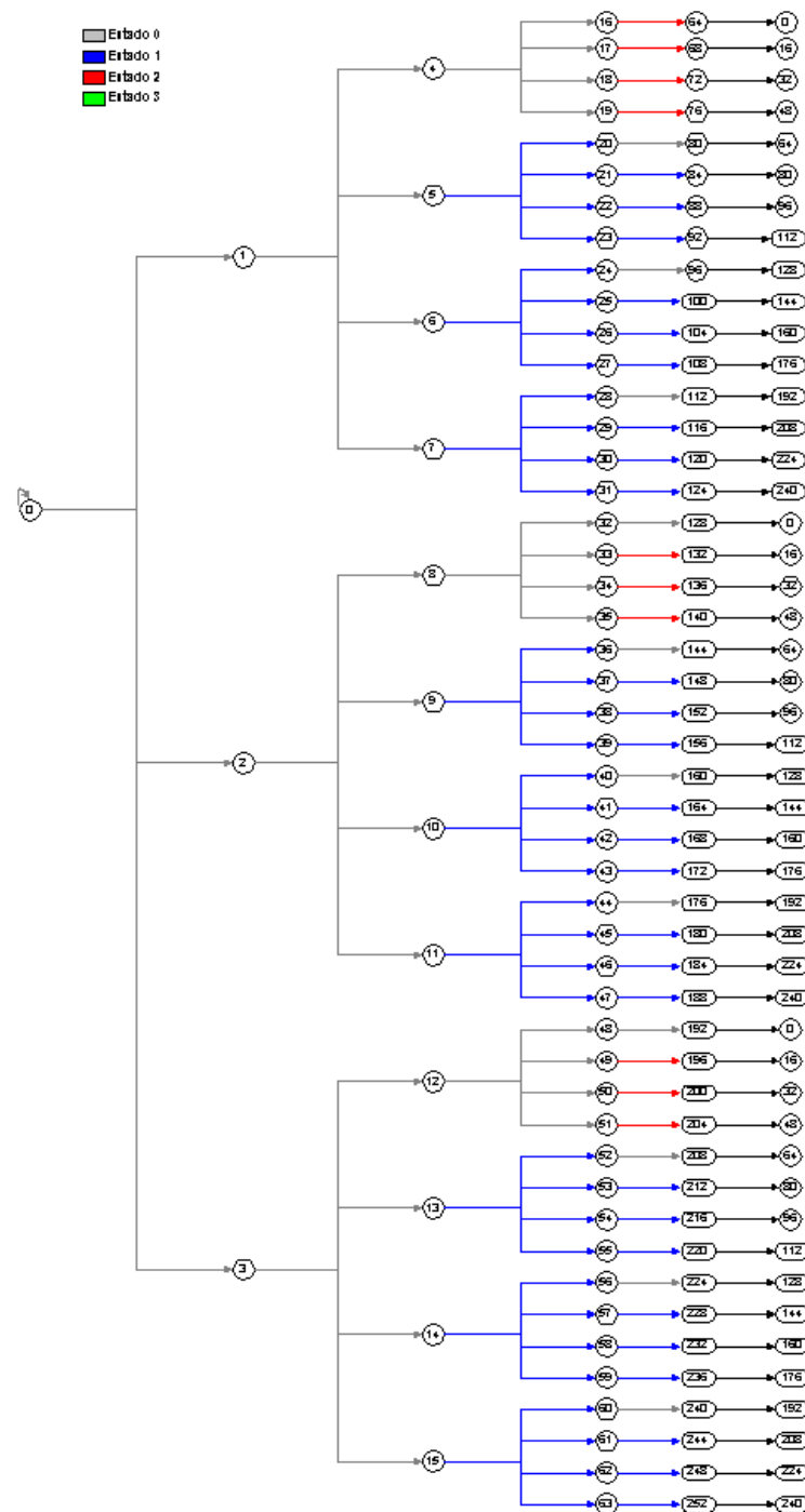
Figura 5.11: Árbol que representa las conexiones entre los nodos del diagrama de Bruijn. En esta figura el árbol está representado de manera resumida. Se puede observar que en algunos casos solo aparecen conectados los nodos que representan el inicio del rango de interconexión.
