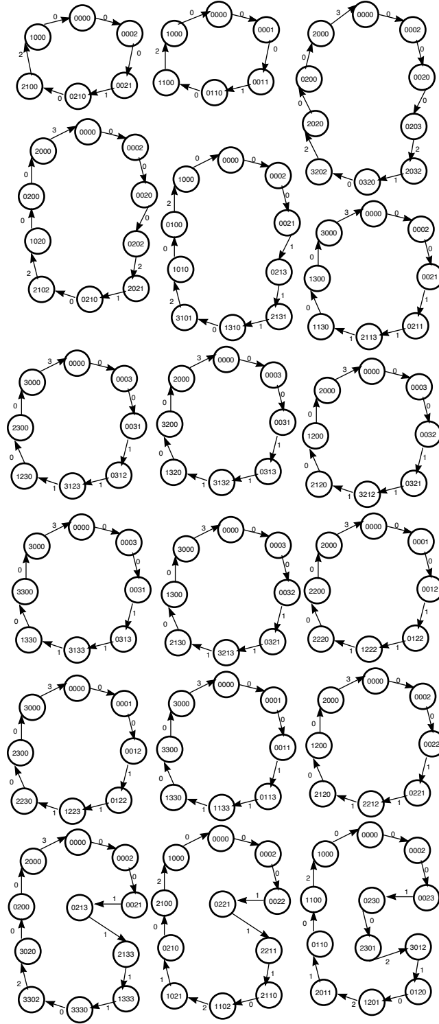
Figura 5.12: Anillos que generan secuencias en las cuales las células no tienen desplazamientos uniformes hacia la derecha.
