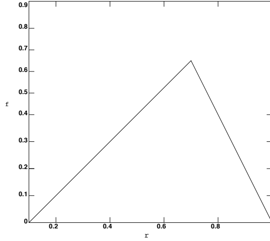
Figura 4.7: Diagrama fundamental del modelo de Fuk s y Boccara.
