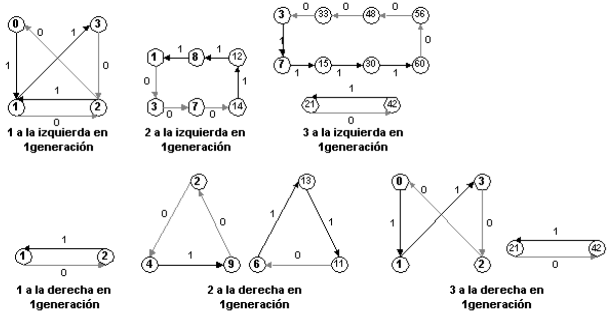
Figura 5.8: Desplazamientos en una generación que tienen las células al aplicar la regla de AC(2,1) 43.
