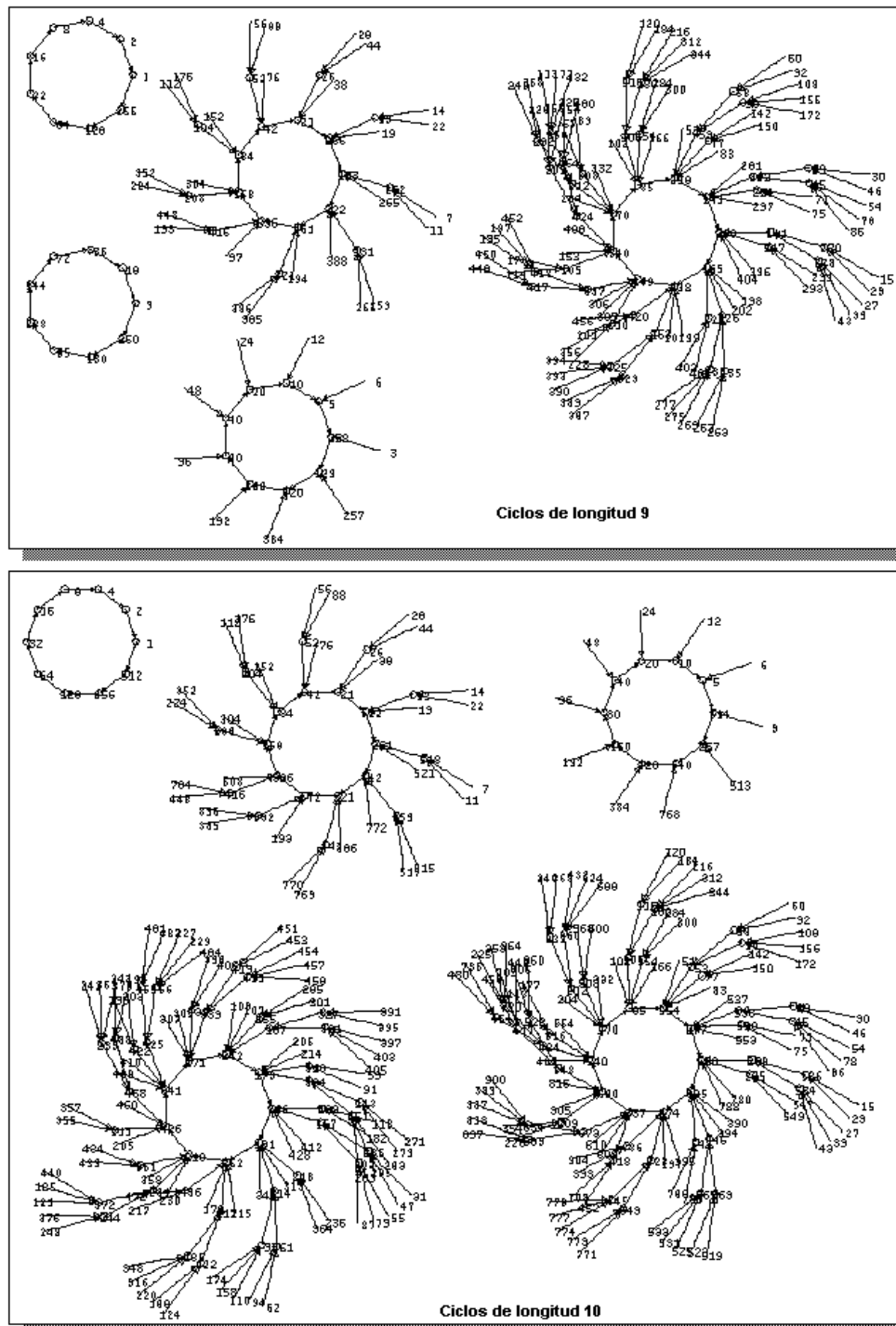
Figura 4.16: Ciclos de periodo 9 y periodo 10 de la regla 184.
