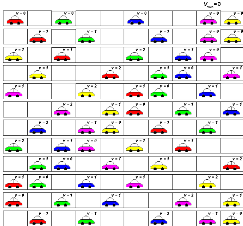
Figura 5.3: Flujo de tránsito de autos aplicando el modelo de Nagel con V_{max} = 3 y \rho = 0.5 .
