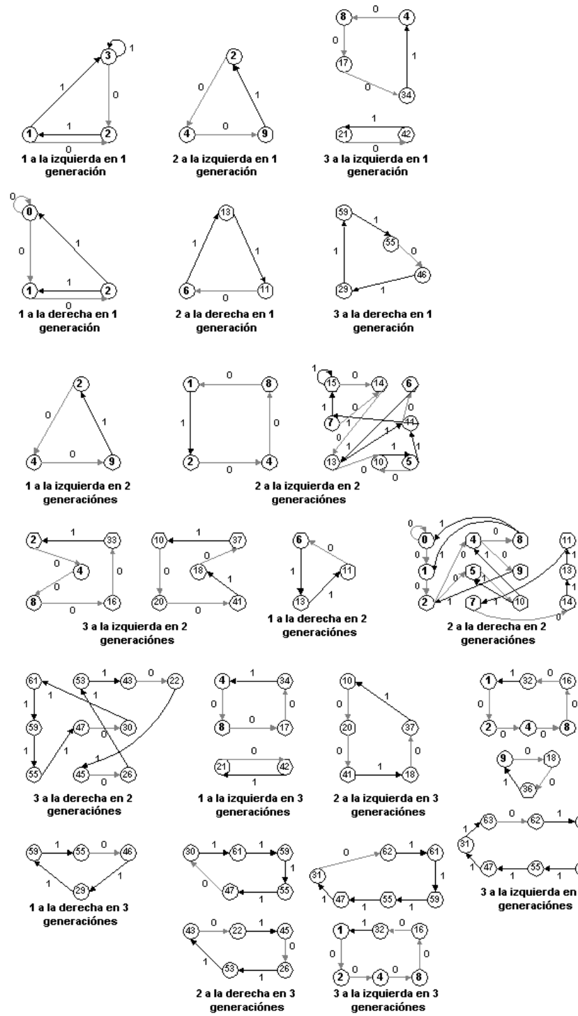
Figura 4.13: Desplazamientos que tienen las células al aplicar la regla de AC(2,1) 184.
