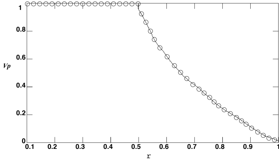
Figura 4.2: Promedio de velocidad de los autos en función de la densidad.
