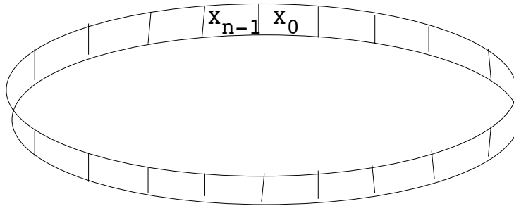
Figura 3.8: Estructura de un autómata celular lineal estableciendo condiciones de límites periódicos.
