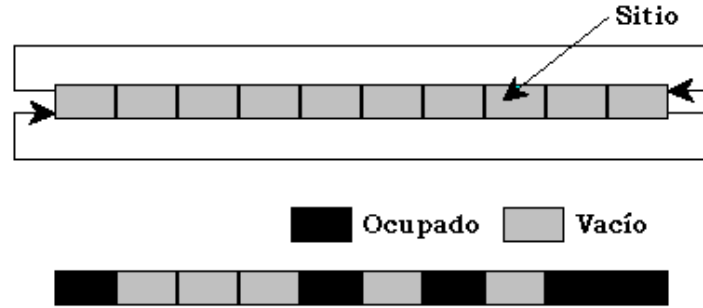
Figura 5.1: Arreglo de 10 sitios.
