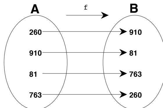
Figura 3.22: Función biyectiva.
