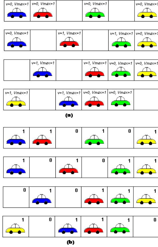
Figura 4.3: (a) Desplazamiento de los autos aplicando el modelo que incluye los parámetros v y V_{max} . (b) Desplazamiento de los autos aplicando la regla de evolución 184 para un AC(2,1).
