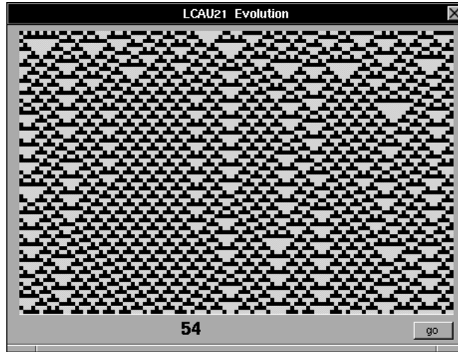
Figura 3.11: Diagrama de evoluciones de un autómata celular lineal (2,1) aplicando la regla 54.
