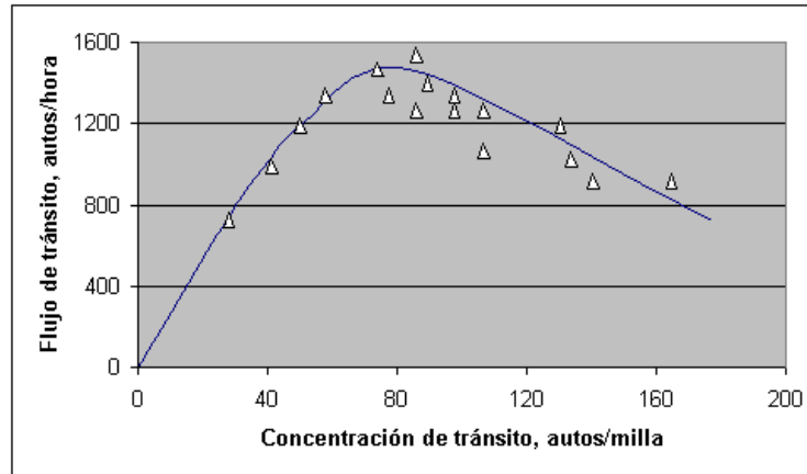
Figura 2.1: Diagrama fundamental de flujo de tránsito.
