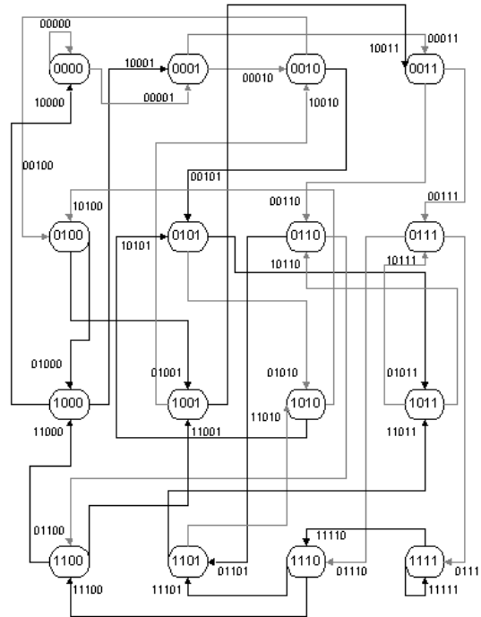
Figura 5.6: Diagrama de Bruijn de la regla 43 extendido a vecindades parciales de 4 células.
