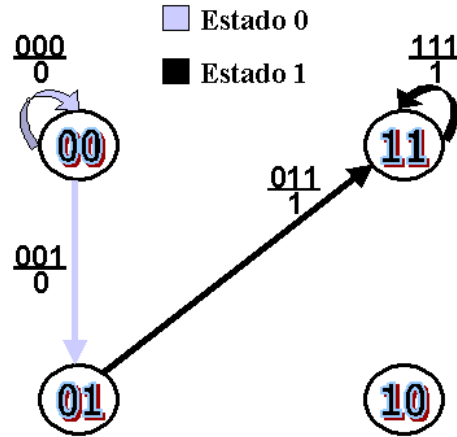
Figura 4.9: Subdiagrama que muestra las configuraciones still lifes de la regla 184.
