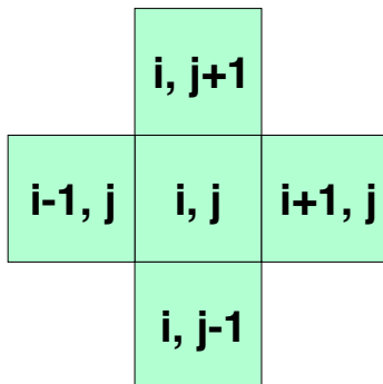
Figura 3.1: Vecindad von Neumann.
