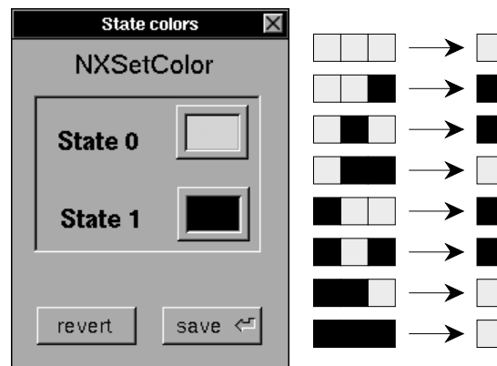
Figura 3.10: Representación de la regla 54 utilizando colores.
