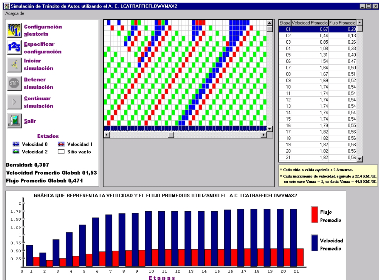
Figura 6.5: Pantalla donde se muestra la evolución del autómata con un arreglo grande.
