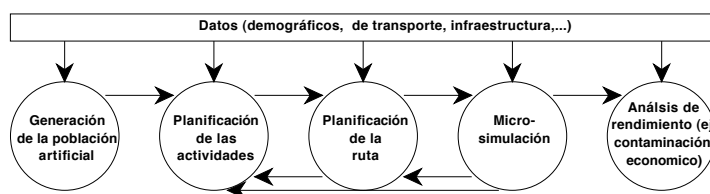
Figura 1.1: Módulos de una simulación basada en agentes que realiza TRANSIMS.
