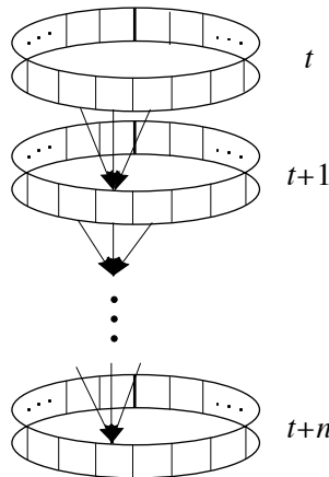
Figura 1.3: Espacio de evoluciones en una dimensión
