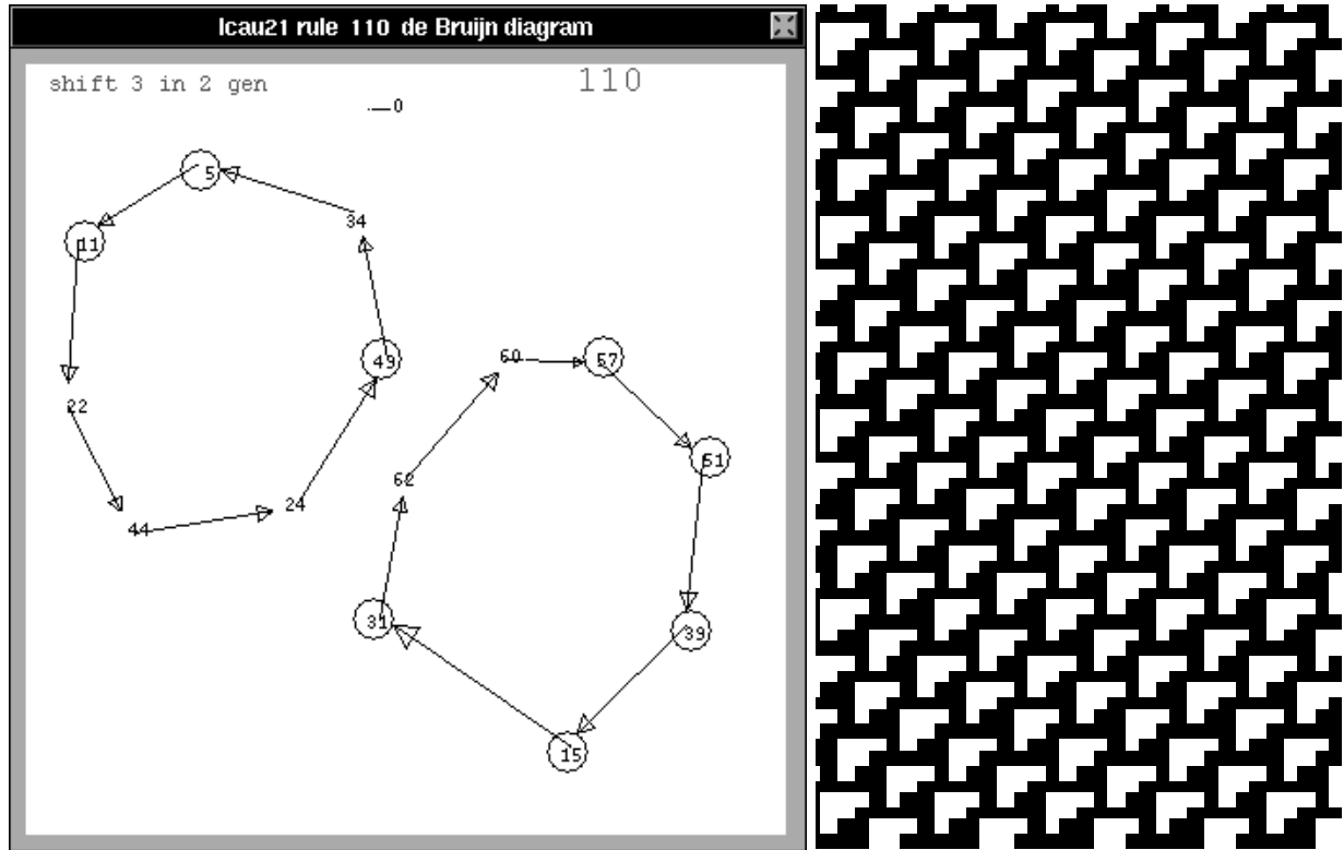
Figura 4.4: Ether en la regla 110
