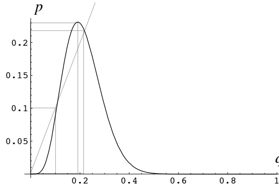
Figura 3.7: Curva de probabilidad de la regla R(4, 5, 5, 5)
