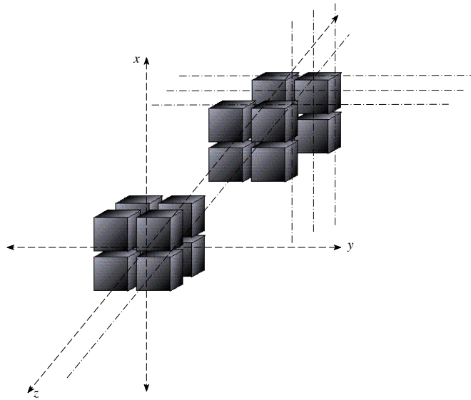
Figura 3.2: Planos adyacentes en tres dimensiones
