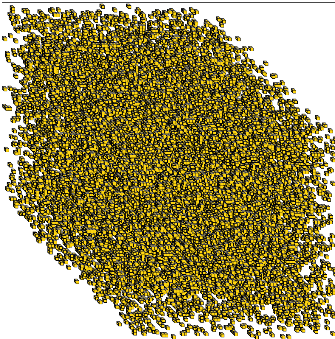
Figura 1.9: Diagrama de evoluciones en tres dimensiones
