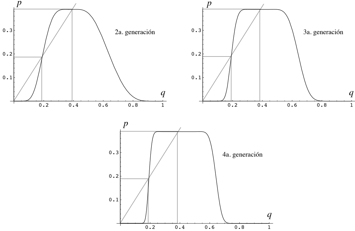
Figura 2.15: Curva de probabilidad de la regla HighLife , segunda, tercera y cuarta generación
