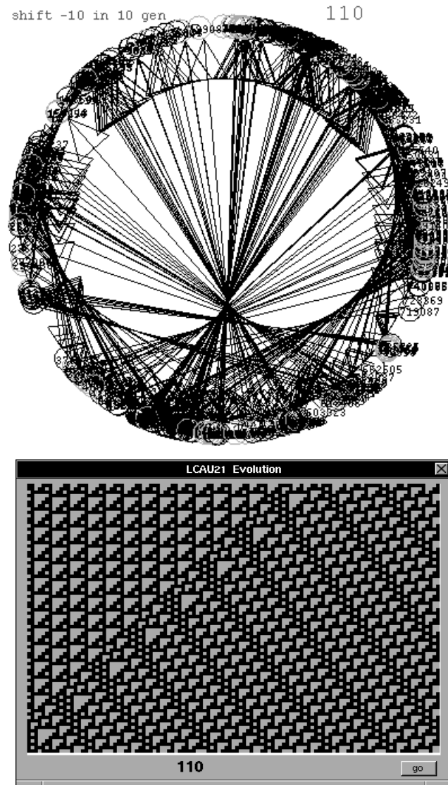
Figura 4.9: Diagrama de de Bruijn extendido en 10 generaciones
