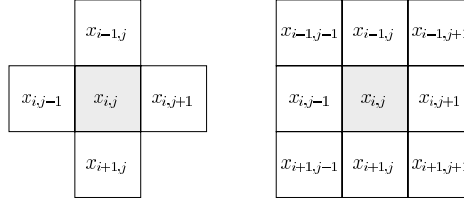
Figura 1.5: Vecindad de von Neumann y vecindad de Moore
