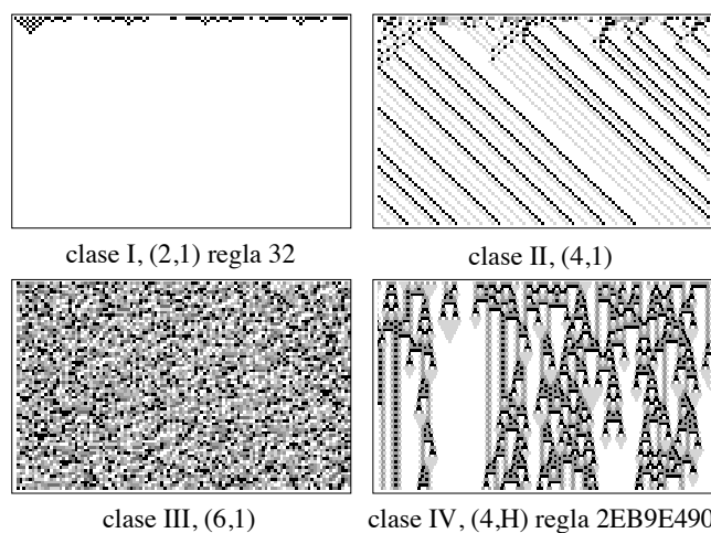
Figura 1.11: Clases de Wolfram
