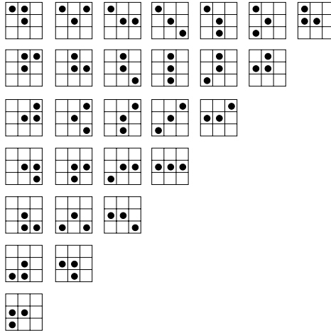
Figura 2.9: Configuraciones que determinan la sobrevivencia cuando S_{min} = 2
