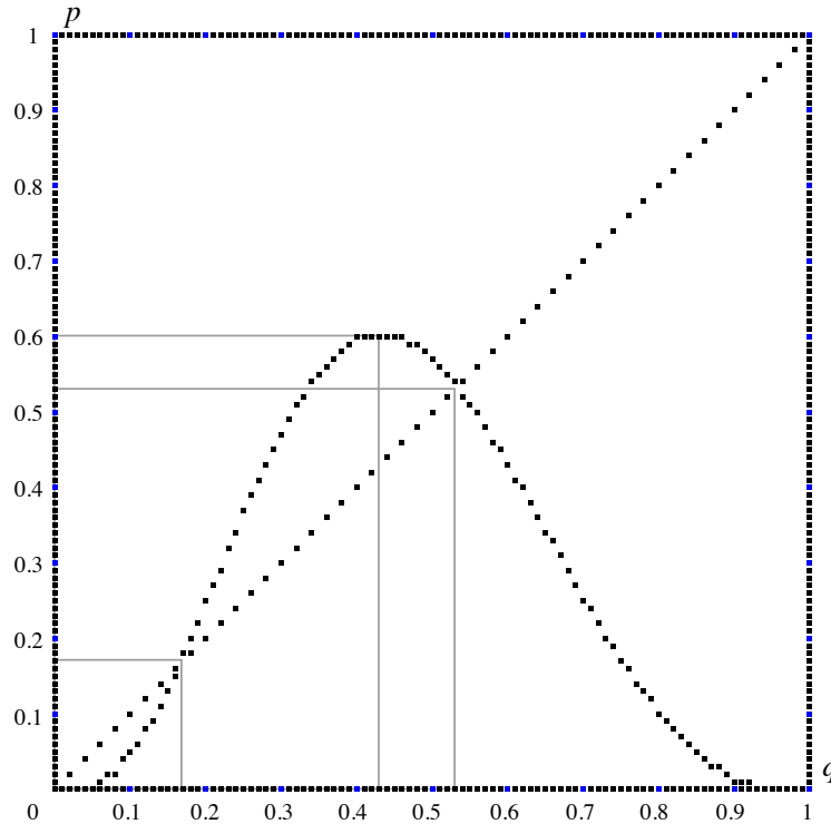
Figura 2.13: Curva de probabilidad de la regla HighLife
