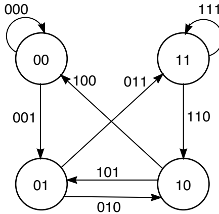
Figura 4.2: Diagrama de de Bruijn genérico (2,1)
