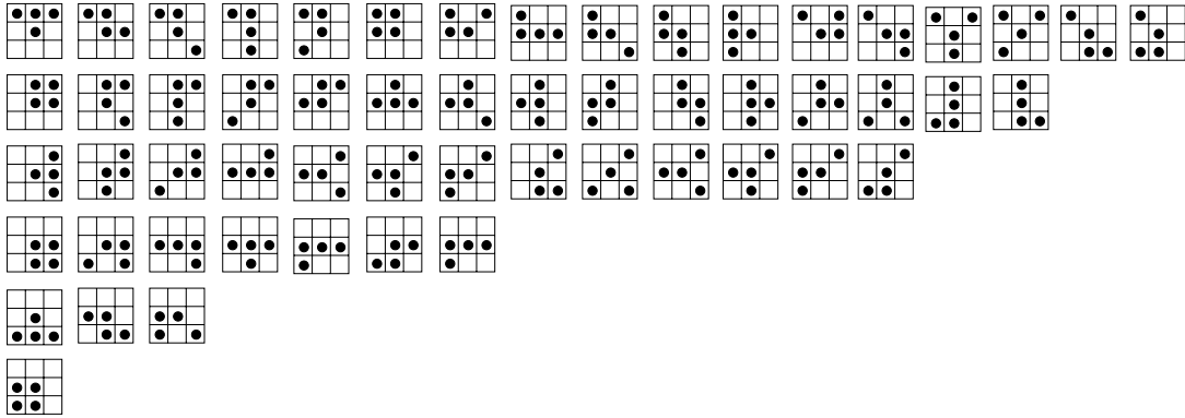
Figura 2.10: Configuraciones que determinan la sobrevivencia cuando S_{max} = 3
