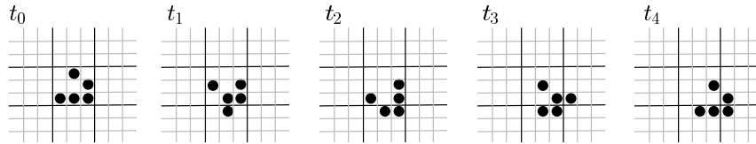
Figura 2.4: Configuración periódica con desplazamiento, glider
