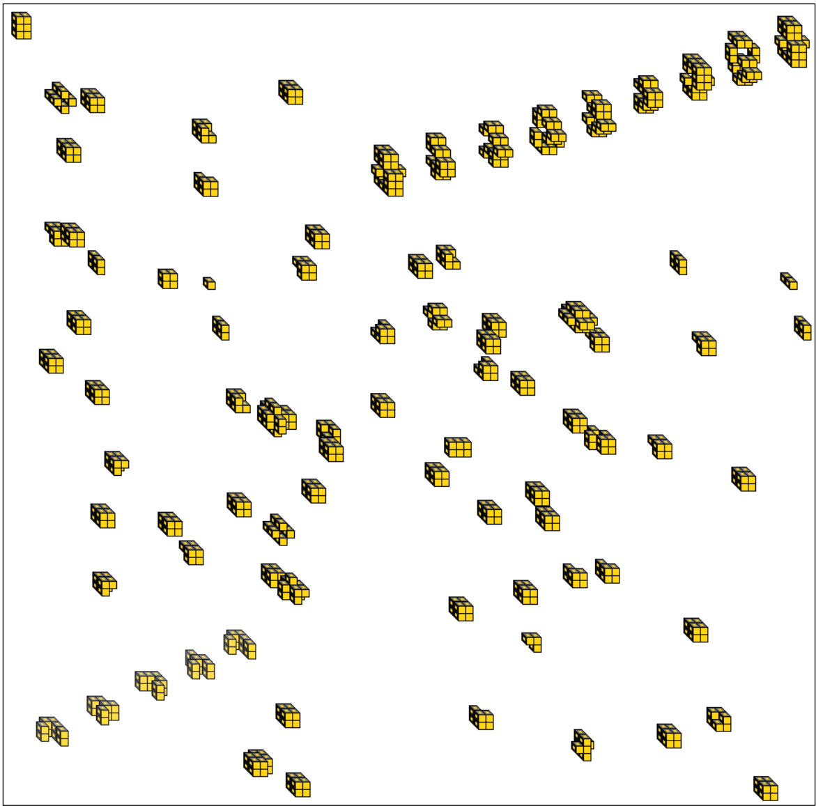
Figura 3.3: Comportamientos de la regla R(5, 7, 6, 6)
