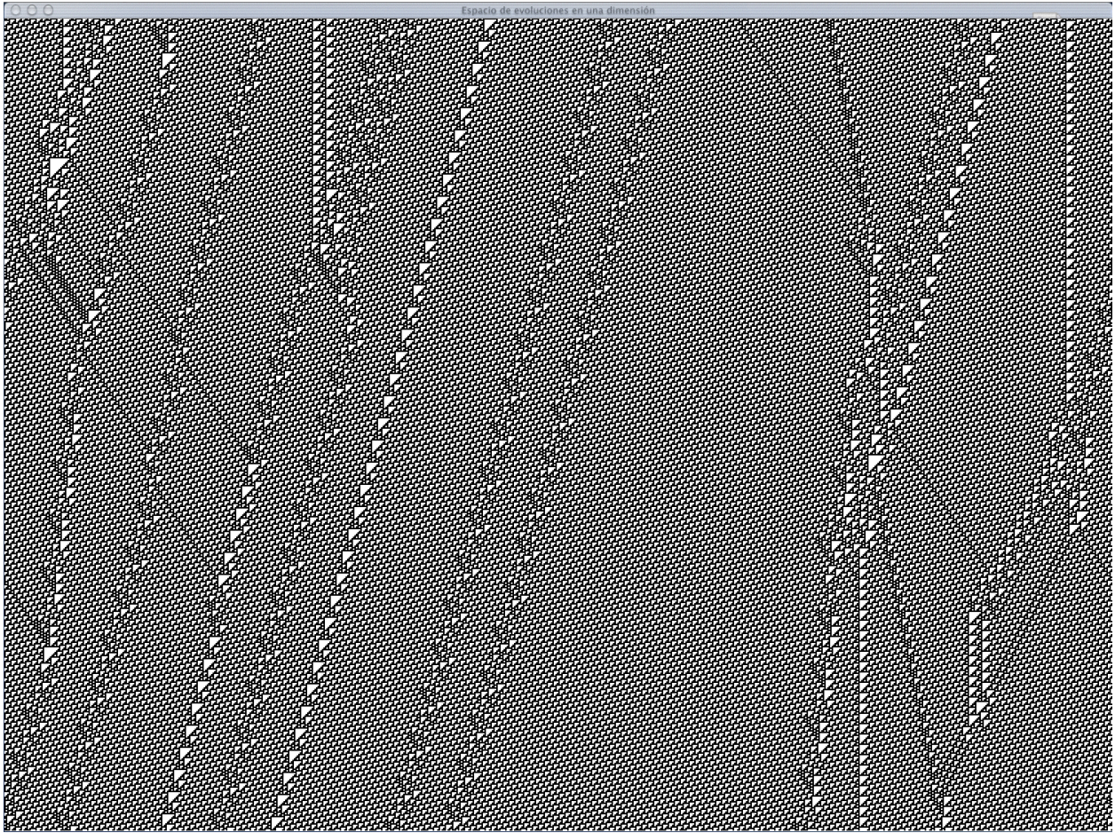
Figura 4.1: Evolución típica de la regla 110
