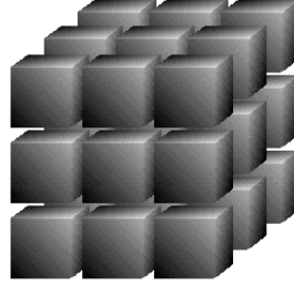
Figura 1.8: Vecindad de Moore en tres dimensiones
