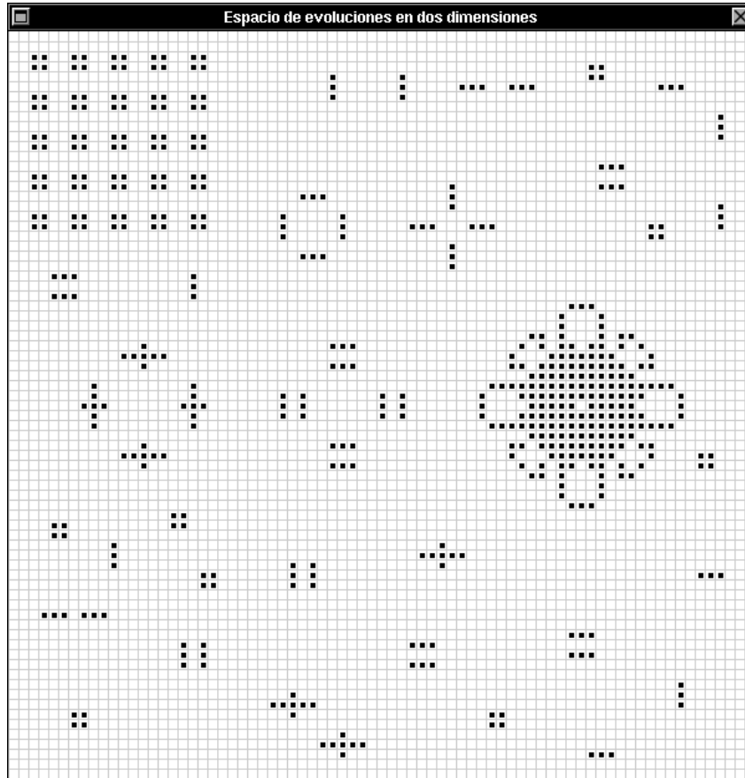
Figura 2.8: Naturaleza muerta y blinkers en HighLife
