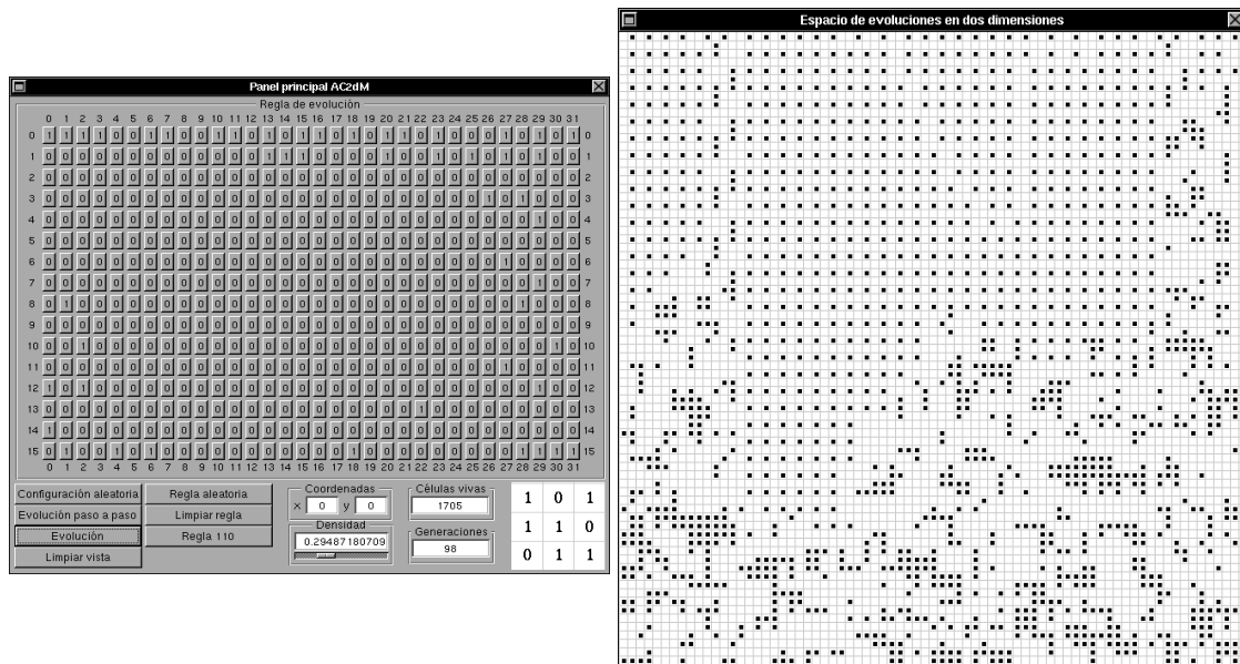
Figura 5.2: Comportamientos complejos empleando vecindad de Moore completa
