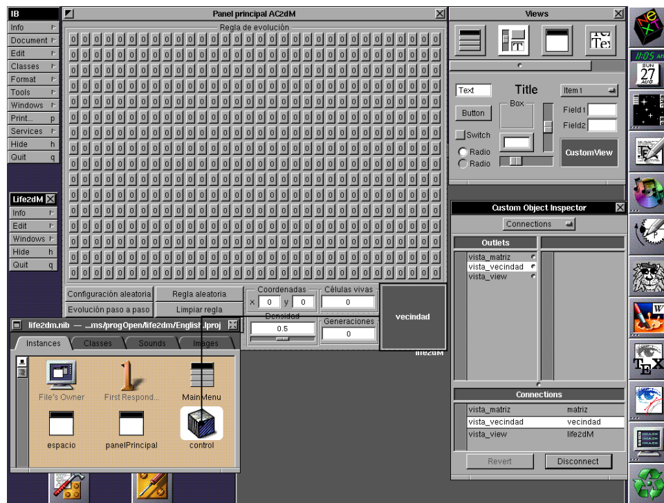
Figura A.11: Conexión de objetos
