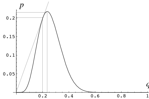
Figura 3.5: Curva de probabilidad de la regla R(5, 7, 6, 6)
