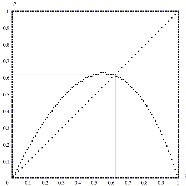
Figura 4.10: Curva de probabilidad de la regla 110
