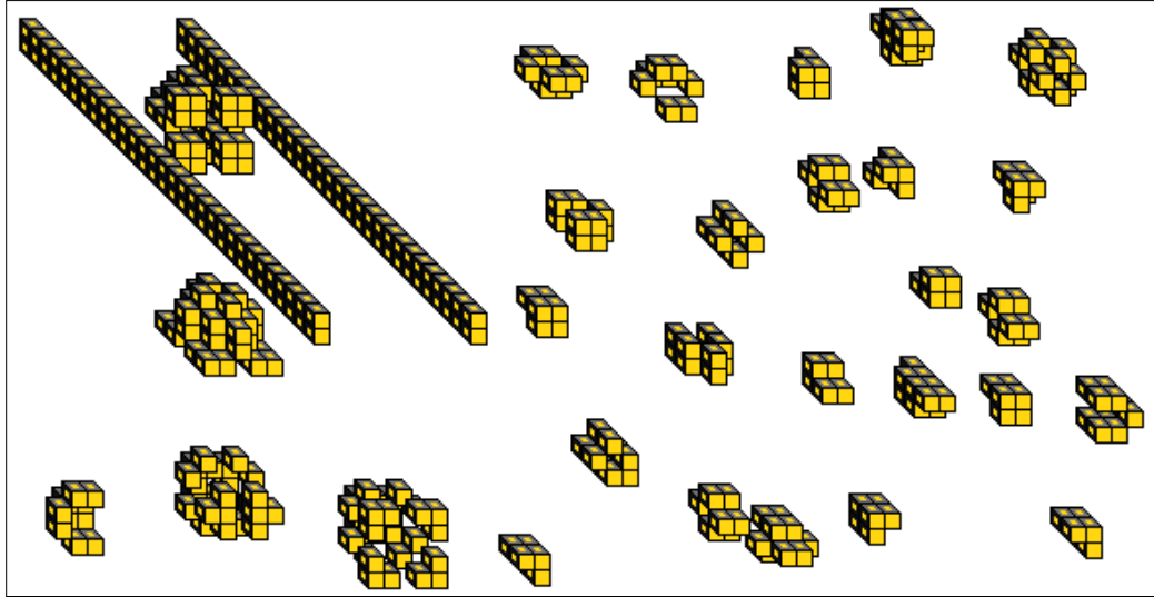
Figura 3.4: Comportamientos de la regla R(4, 5, 5, 5)
