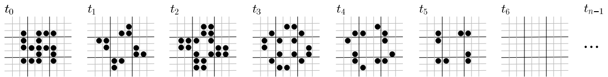
Figura 2.1: Configuración que desaparece, estructura swastika
