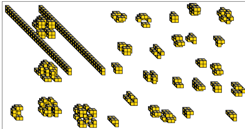
Figura 1.10: Evoluciones en tres dimensiones regla R(4, 5, 5, 5)
