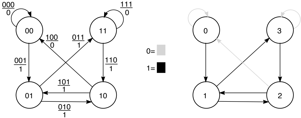
Figura 4.3: Diagrama de de Bruijn para la regla 110
