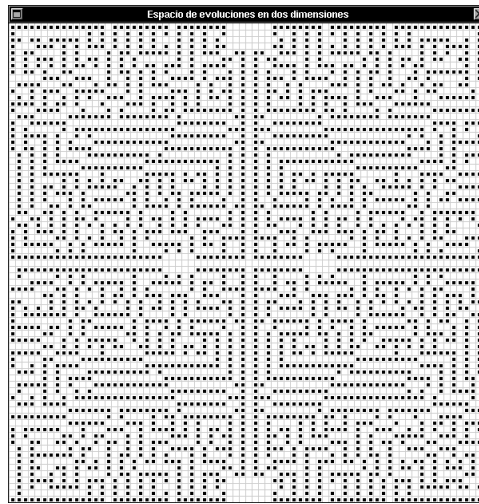
Figura 5.1: Regla semitotalística R(2,4,3,3) empleando vecindad de Moore
