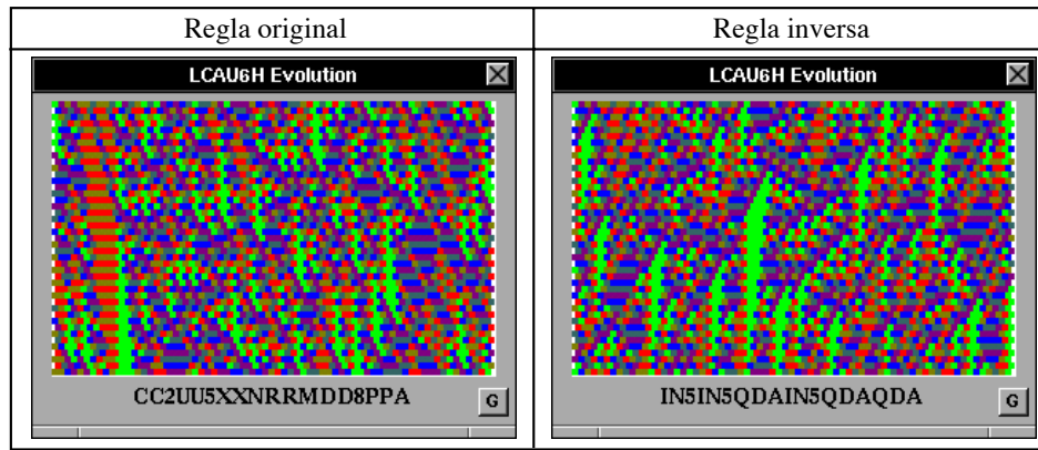
Figura 1.12: Autómata celular reversible en una dimensión
