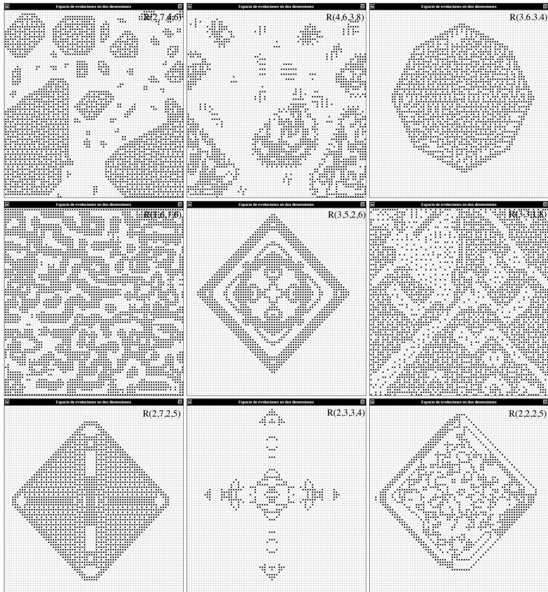
Figura 2.16: Reglas complejas en dos dimensiones
