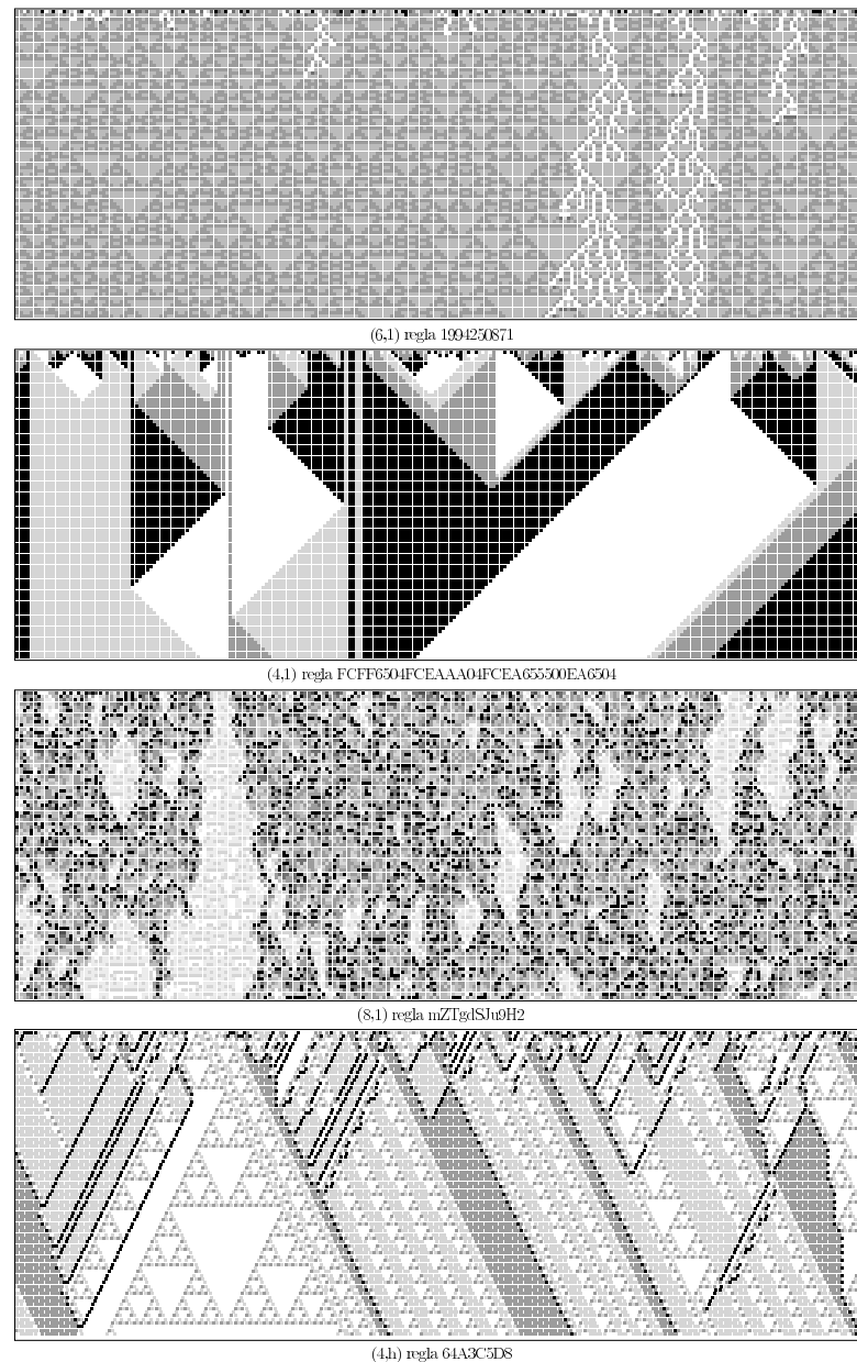
Figura 1.16: Autómatas celulares de clases no definidas
