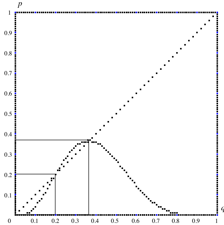
Figura 2.11: Curva de probabilidad de la regla Life
