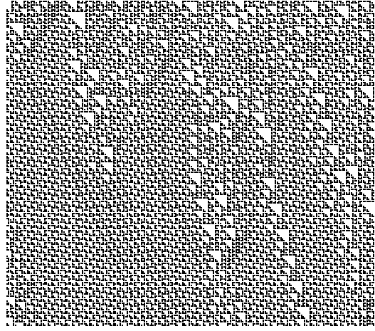
Figura 1.4: Diagrama de evoluciones en una dimensión regla 124
