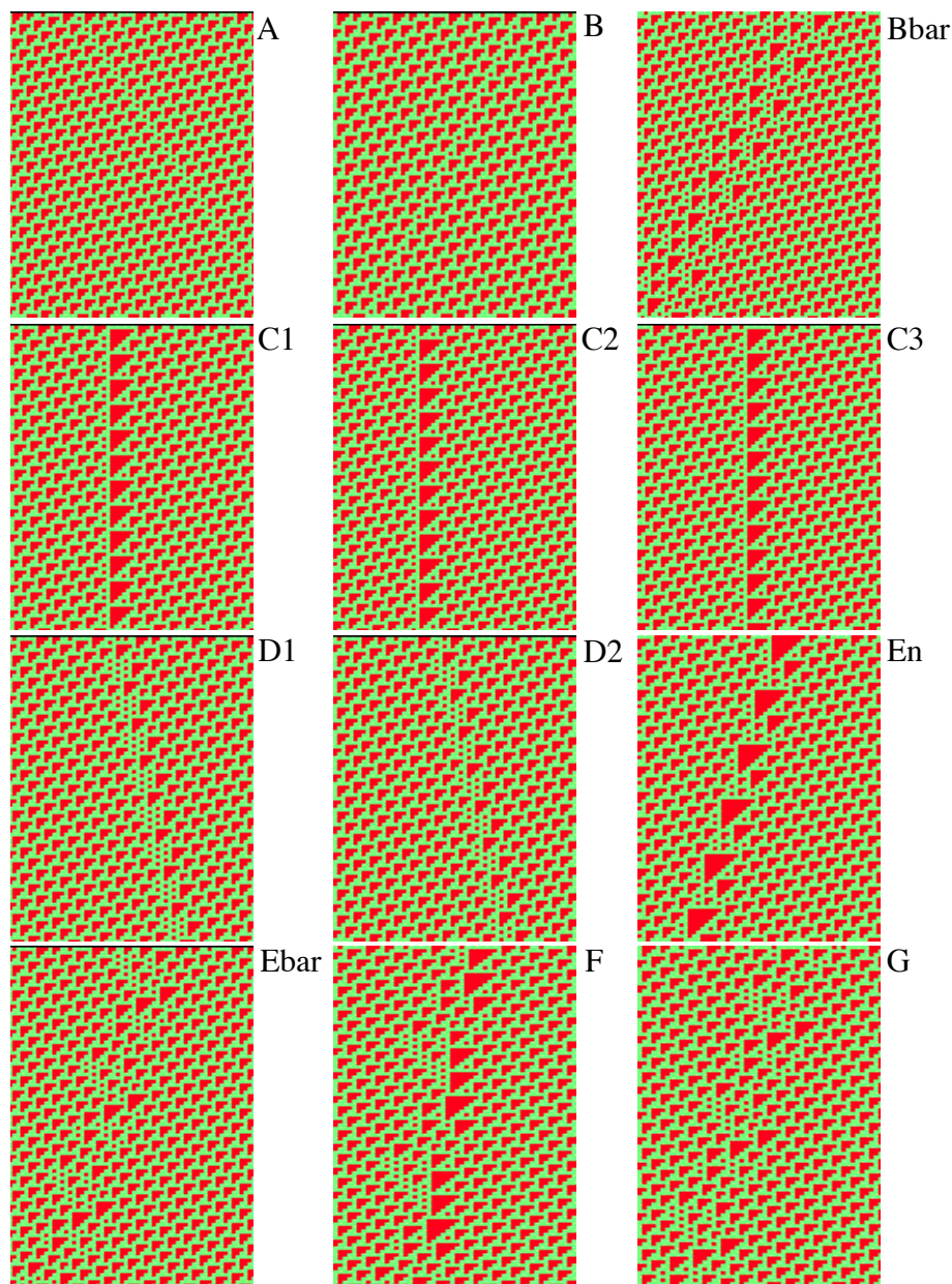
Figura 4.8: Algunos gliders de la regla 110
