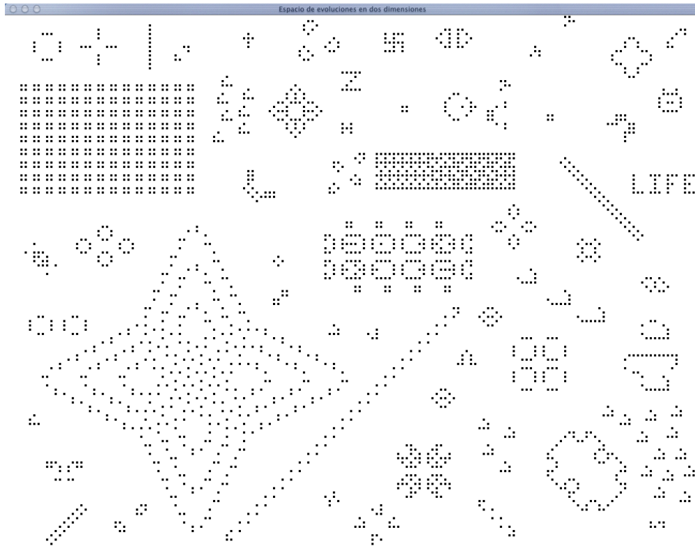
Figura 1.7: Configuraciones complejas en Life
