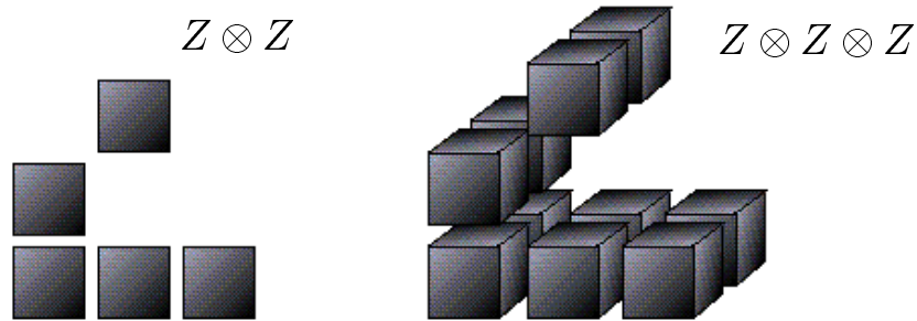
Figura 3.1: Expansiones de Life en tres dimensiones
