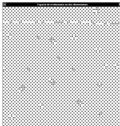
Figura 5.4: Regla semitotalística R(2, 2, 2, 4) empleando vecindad de von Neumann.
