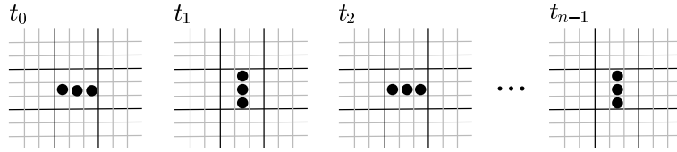
Figura 2.3: Configuración periódica, estructura periódica blinker
