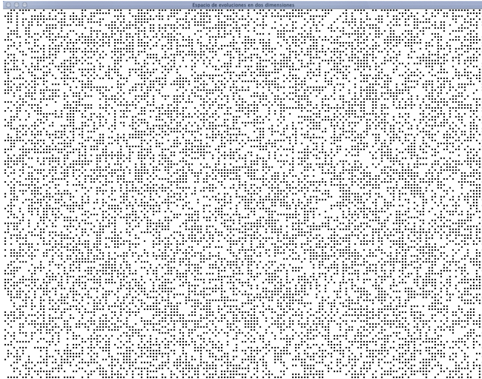
Figura 1.6: Espacio de evoluciones en dos dimensiones
