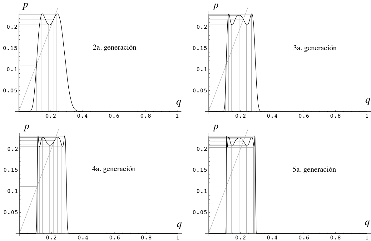
Figura 3.8: Curvas de probabilidad de la regla R(4, 5, 5, 5) segunda, tercera, cuarta y quinta generación
